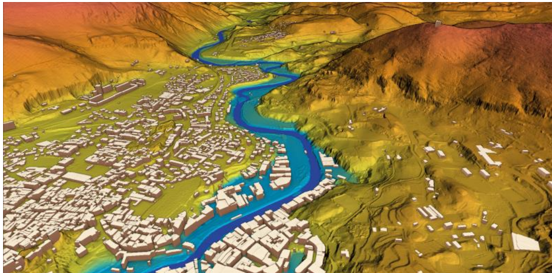
Image de Lourdes issue du programme LiDAR HD montrant le Gave de Pau dans son lit (en bleu foncé, 373 mètres d'altitude) et la zone basse à proximité de la rivière qui pourrait subir des inondations sur certaines zones (en bleu clair, 377 mètres d'altitude). Les modèles des bâtiments ont été ajoutés. © IGN
